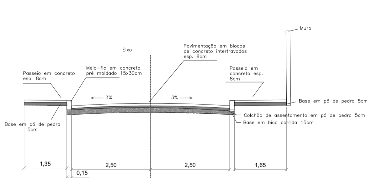
PERFIL D-D
