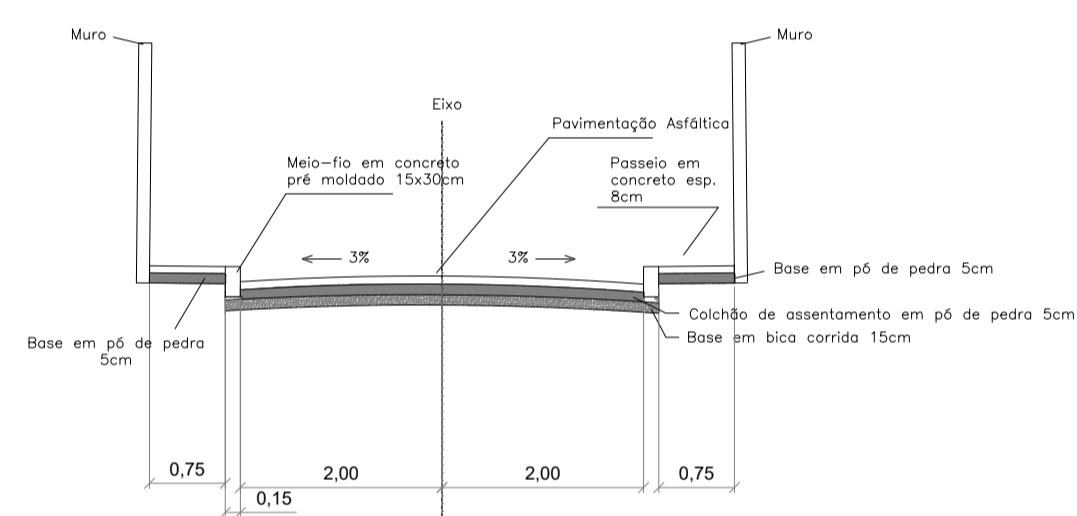
PERFIL B-B
