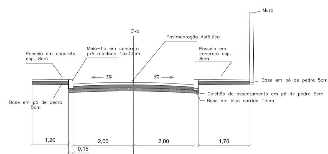
PERFIL A-A
