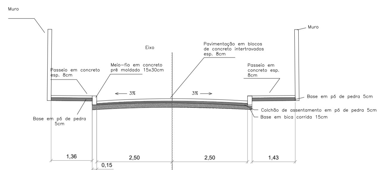
PERFIL C-C
